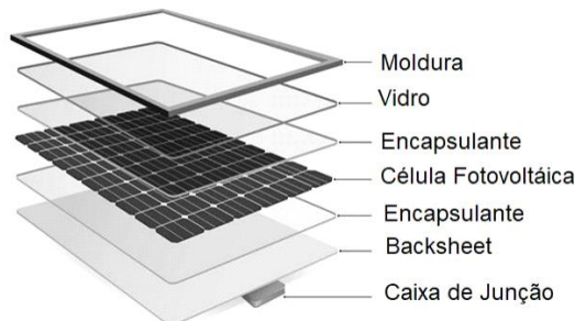
Figura 1: Característica construtiva de um módulo fotovoltaico
