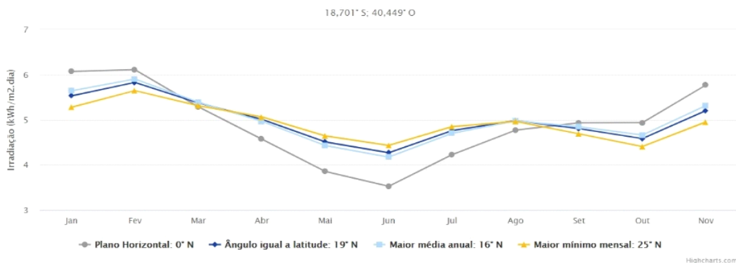
Irradiação Solar no Plano Inclinado –Nova Venecia–Nova Venecia, ES–BRASIL
